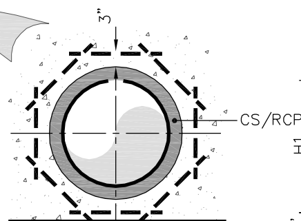
ADD'L PIPE REINFORCING
